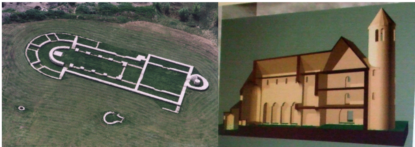
KPôdorys baziliky v Zalaváre (Blatnohrade) a jej 3D rekonštrukcia
